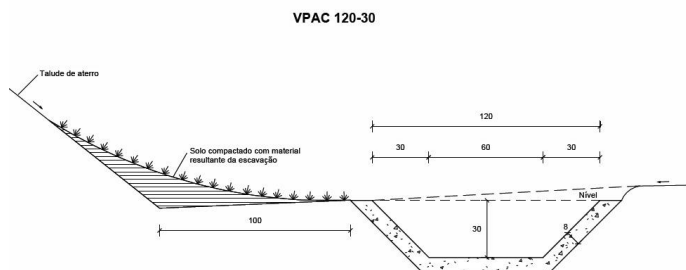
Figura 2 - Valeta de proteção de aterros com revestimento de concreto - VPAC 120-30
