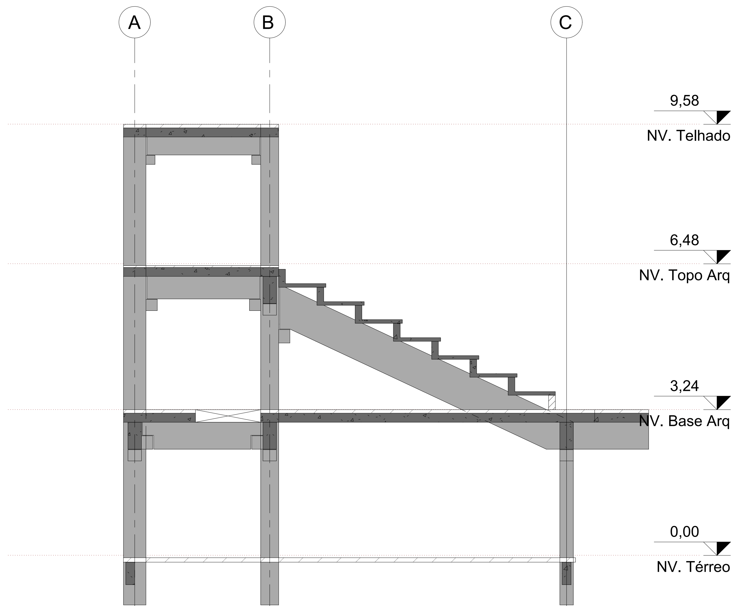
CORTE C-C
