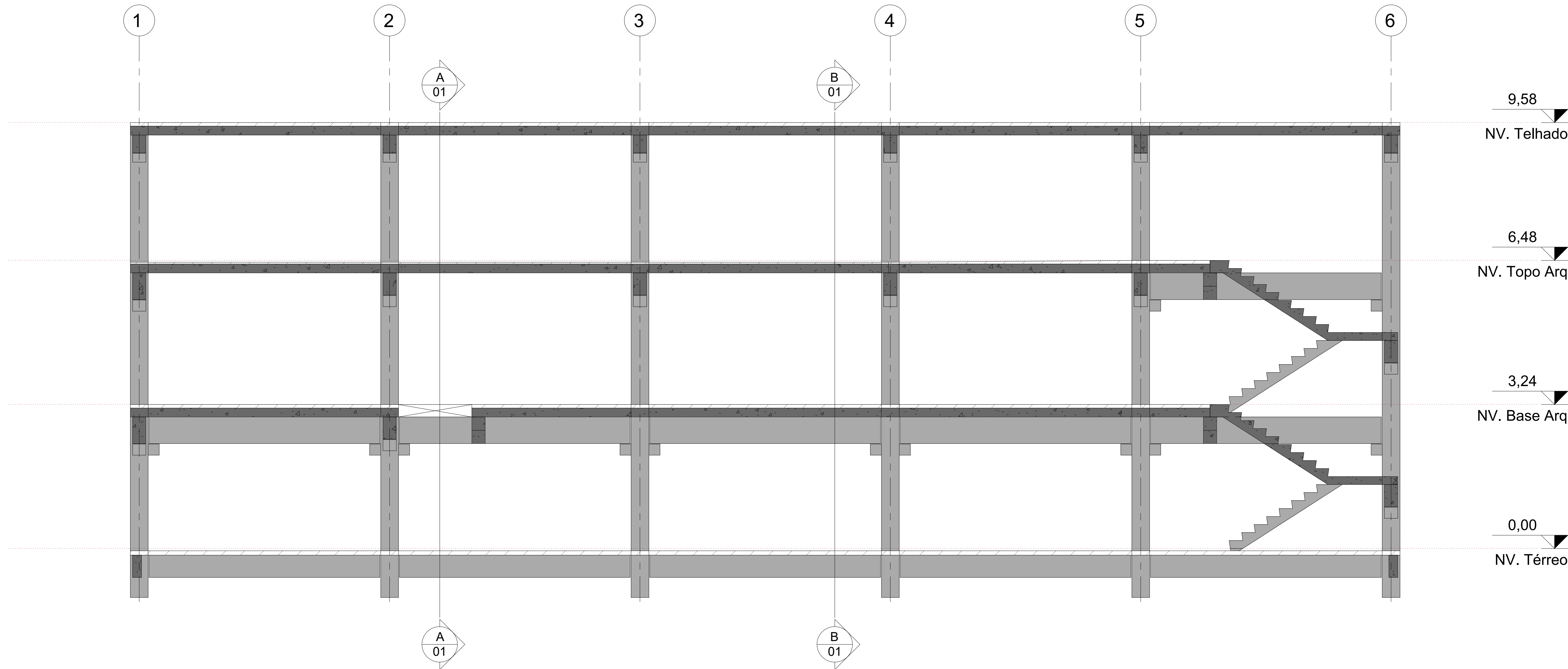
CORTE C-C
