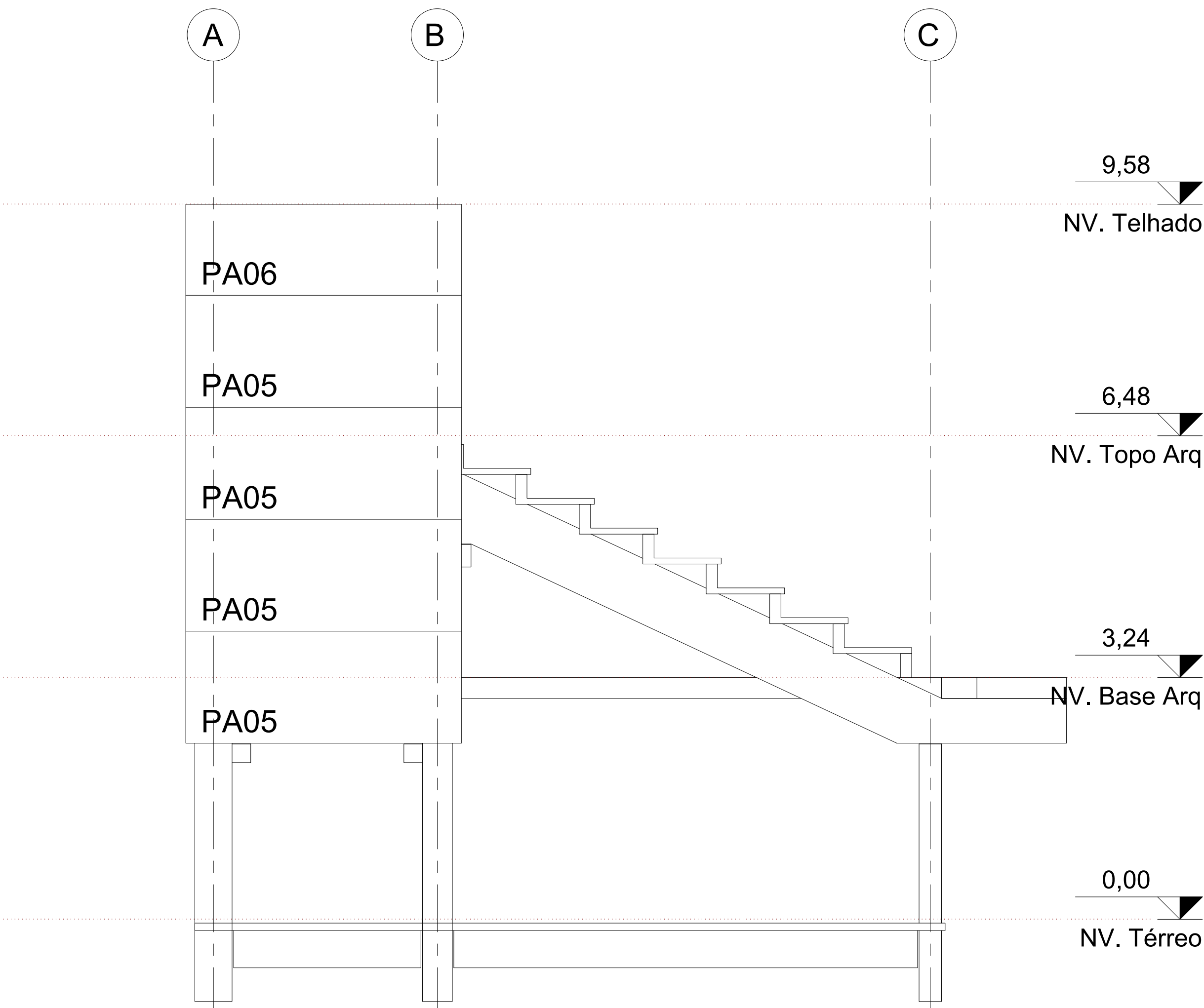
FACHADA LATERAL DIREITA ESC: 1/50
