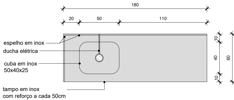
VISTA SUPERIOR BANCADA COM PIA - SALAS 8 E 10 Esc. 1/25
