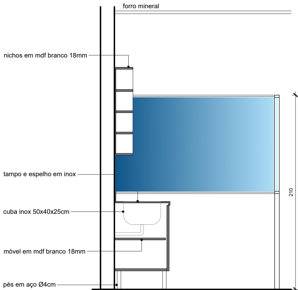
VISTA B - SALA 8 E 10 Esc. 1/25
