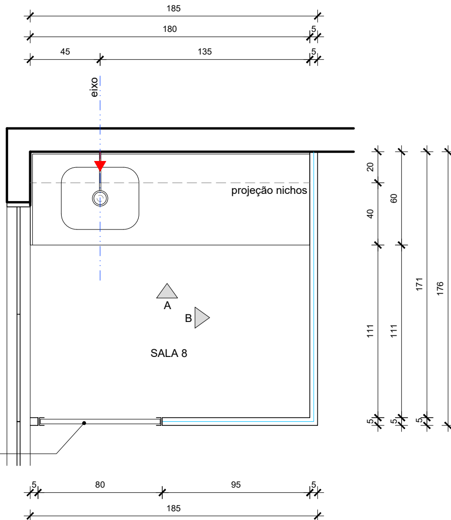
PLANTA BAIXA - SALA 8 Esc. 1/25
