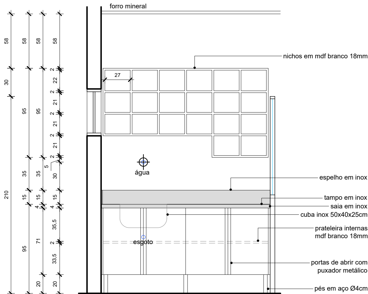
VISTA A - SALAS 8 E 10 Esc. 1/25
