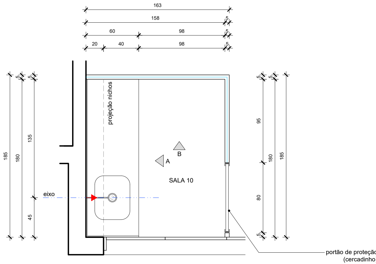
PLANTA BAIXA - SALA 10 Esc. 1/25
