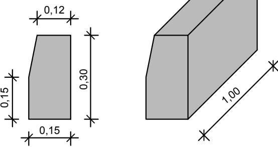
MEIO-FIO DE CONCRETO
