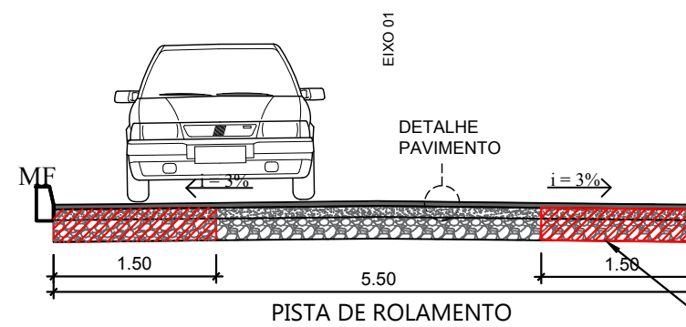
SEÇÃO TIPO DE PAVIMENTO - PAVS CORTE AA'
