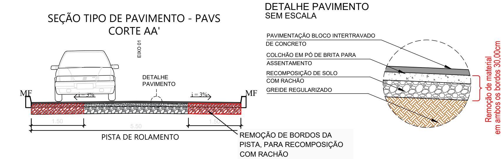
PROJETO GEOMÉTRICO ESCALA: 1/500
