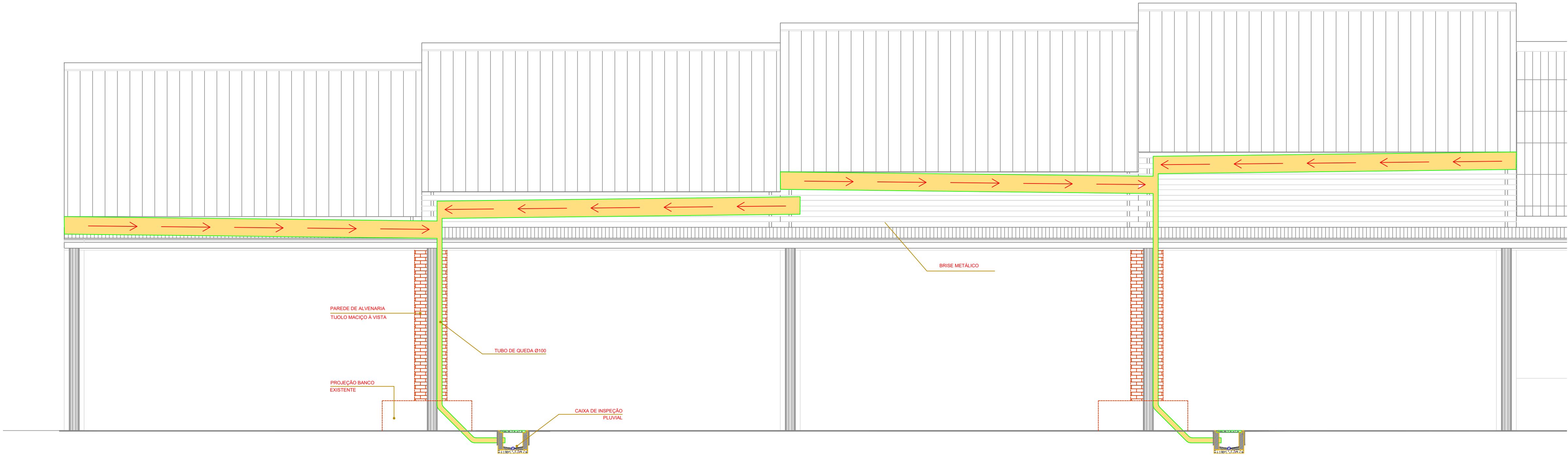
LAYOUT ORIENTAÇÃO CALHAS NOVAS esc 1:50
