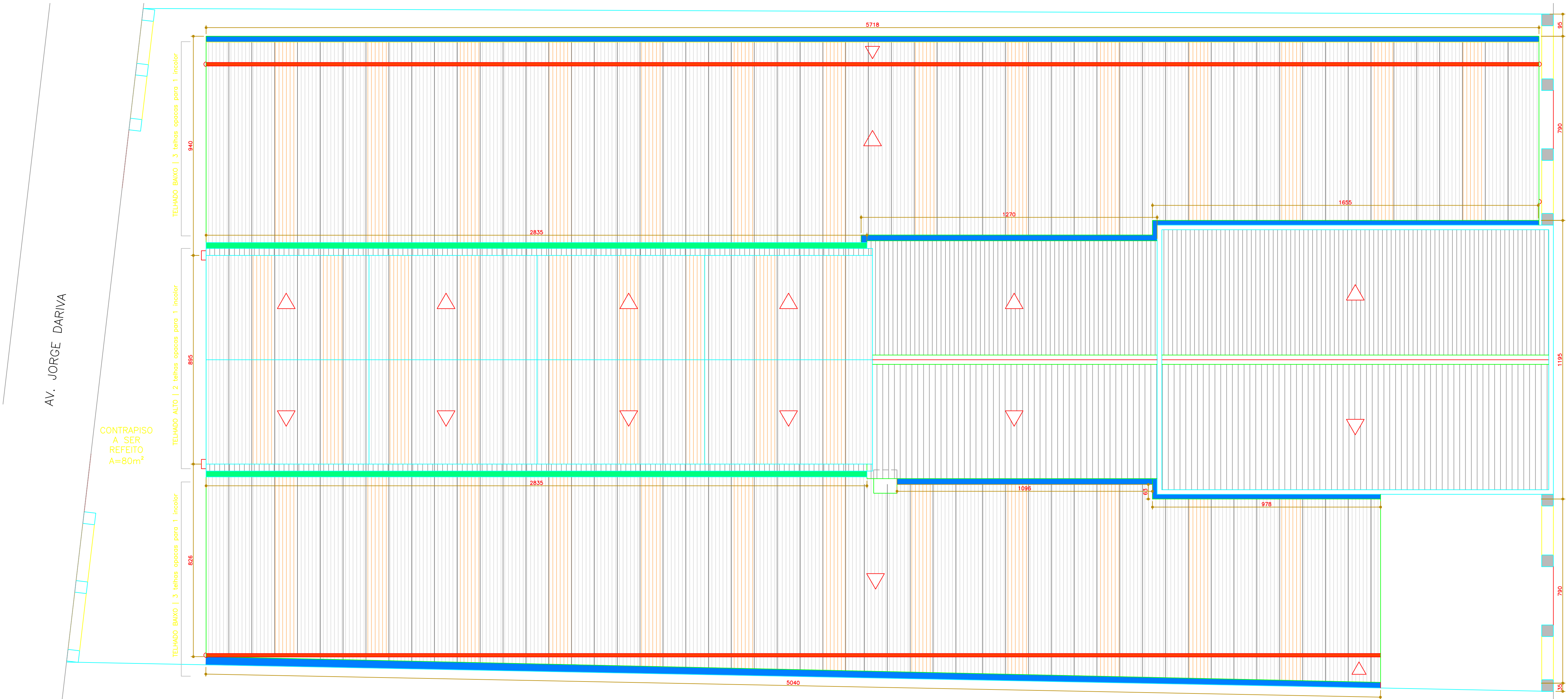
PLANTA BAIXA esc 1:100
