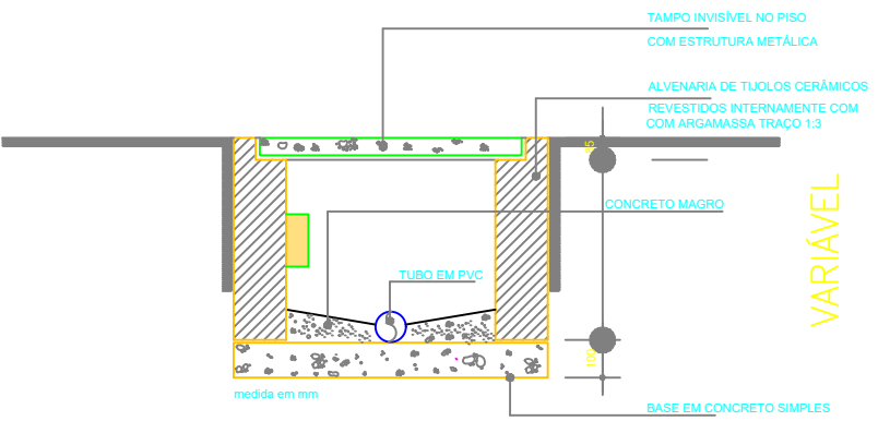
DETALHE CAIXA PLUVIAL esc 1:25
