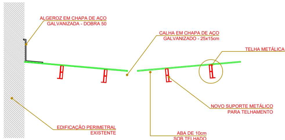
DETALHE CALHA A SER REFORMADA esc 1:25
