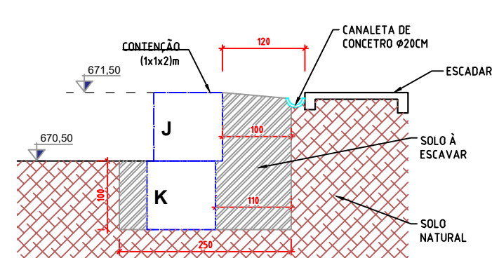
Corte J
