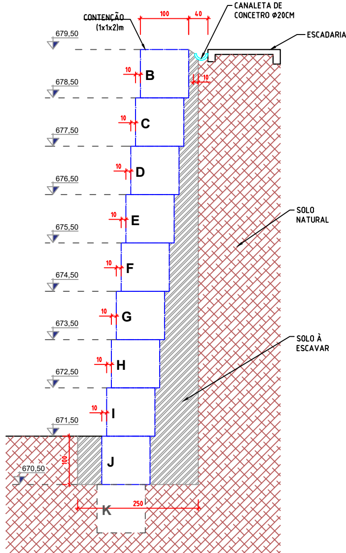
Corte B
