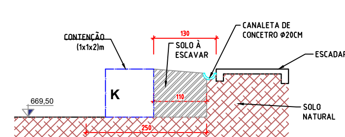
Corte K
