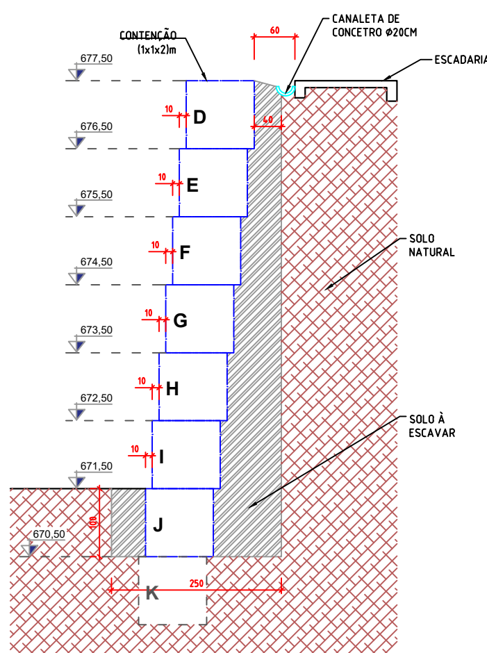
Corte D
