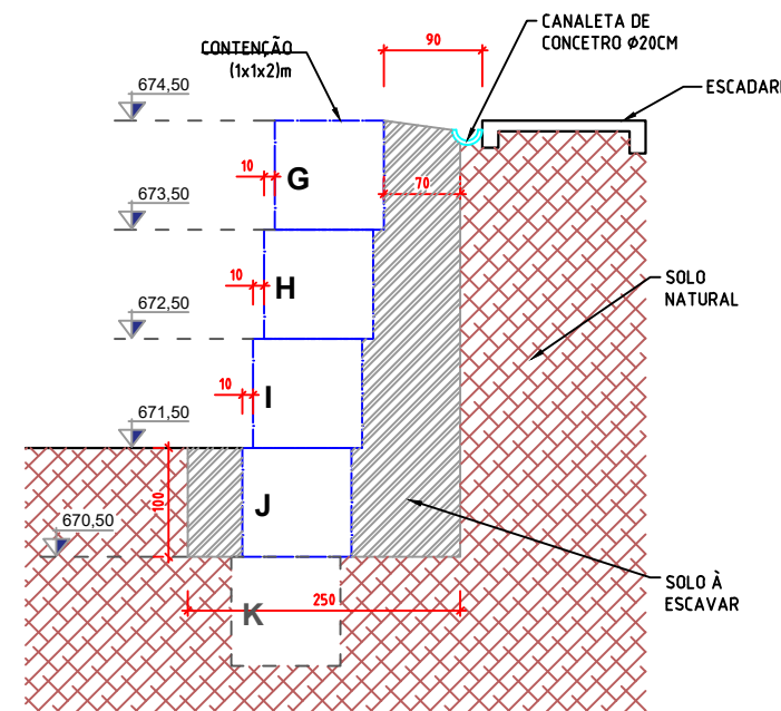
Corte G
