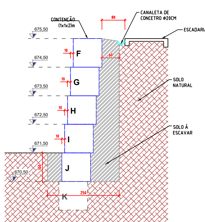
Corte F
