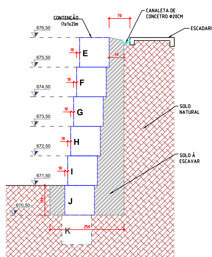
Corte E
