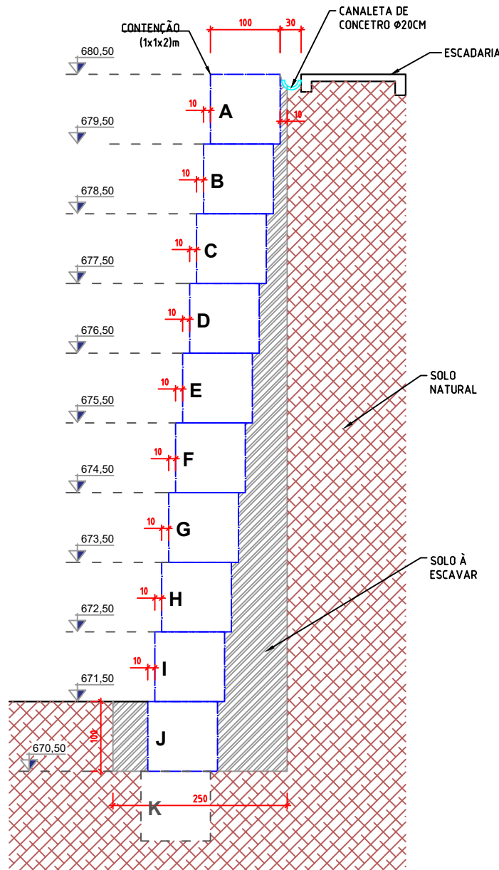
Corte A
