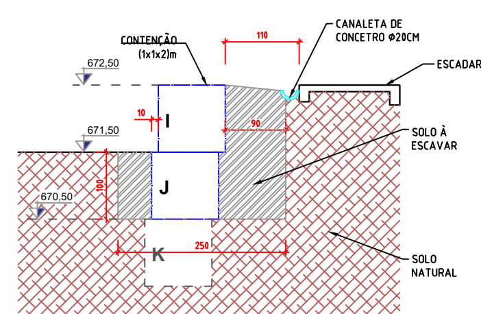
Corte I
