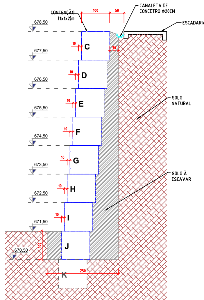
Corte C
