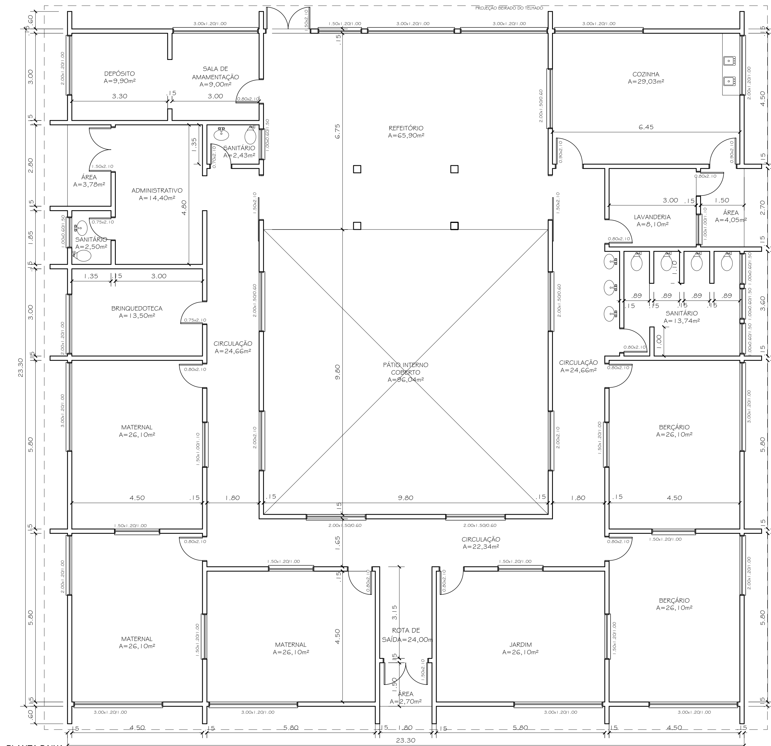
PLANTA BAIXA Esc.: 1/75
