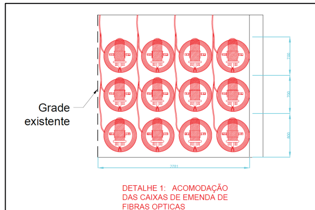
FIGURA 2 - DETALHE DE ACOMODAÇÃO DAS CAIXAS DE EMENDAS ÓPTICAS
