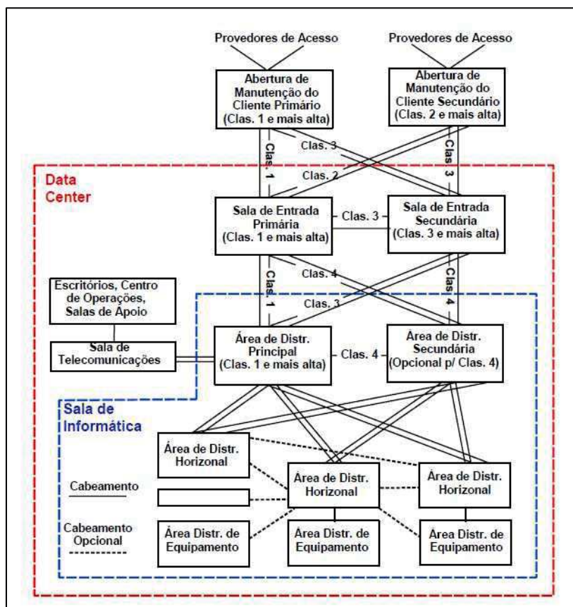
FIGURA 3 - REDUNDÂNCIA DE INFRAESTRUTURA DE COMUNICAÇÃO - FONTE: ANSI/TIA 942
