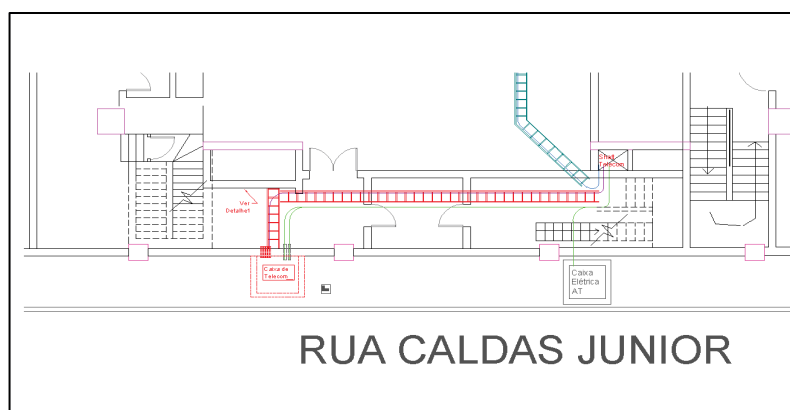
FIGURA 1 - ENTRADA DE CABOS TELECOM NO SUBSOLO DO ED. BANRISUL
