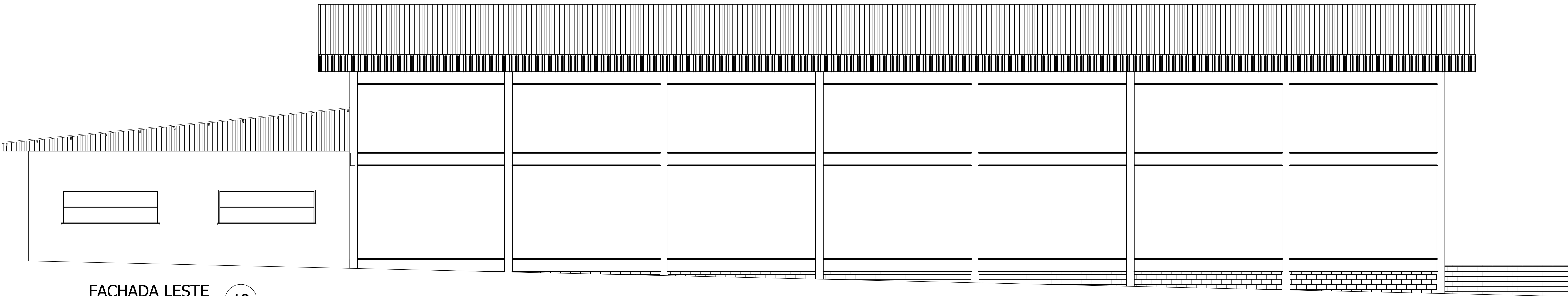
FACHADA LESTE escala: 1:50
