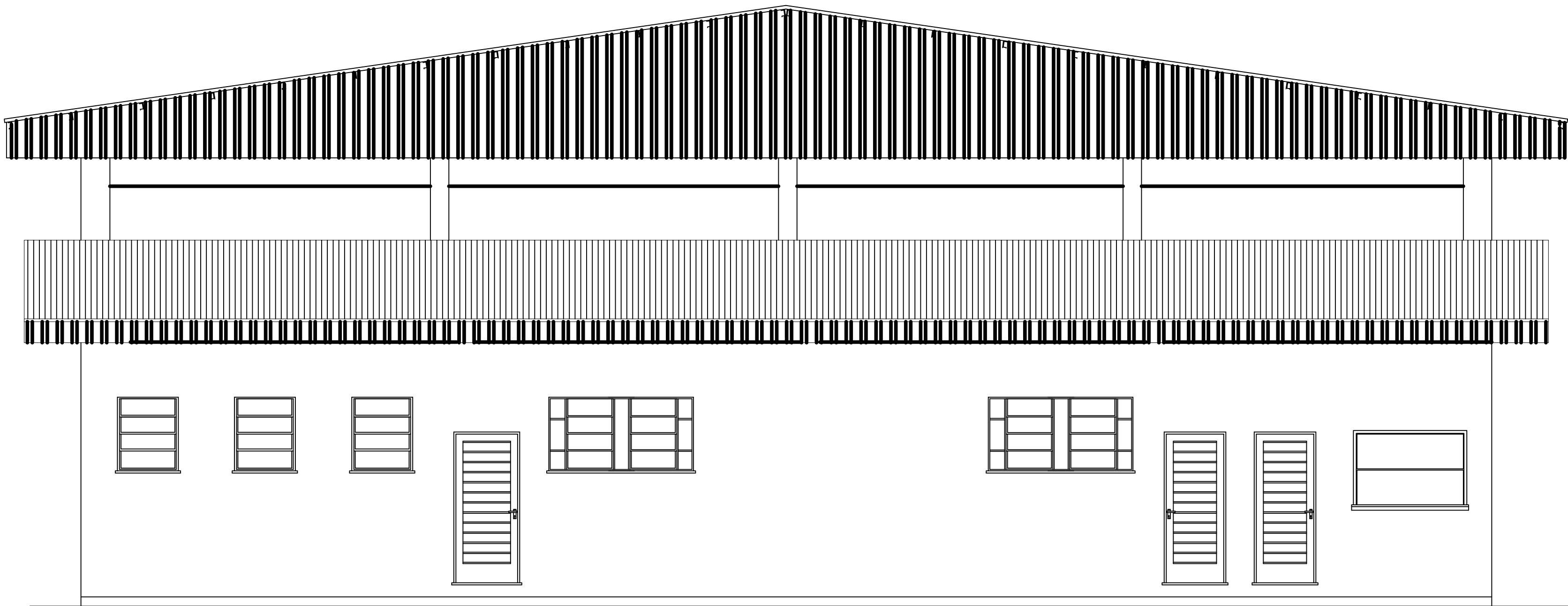
FACHADA NORTE escala: 1:50
