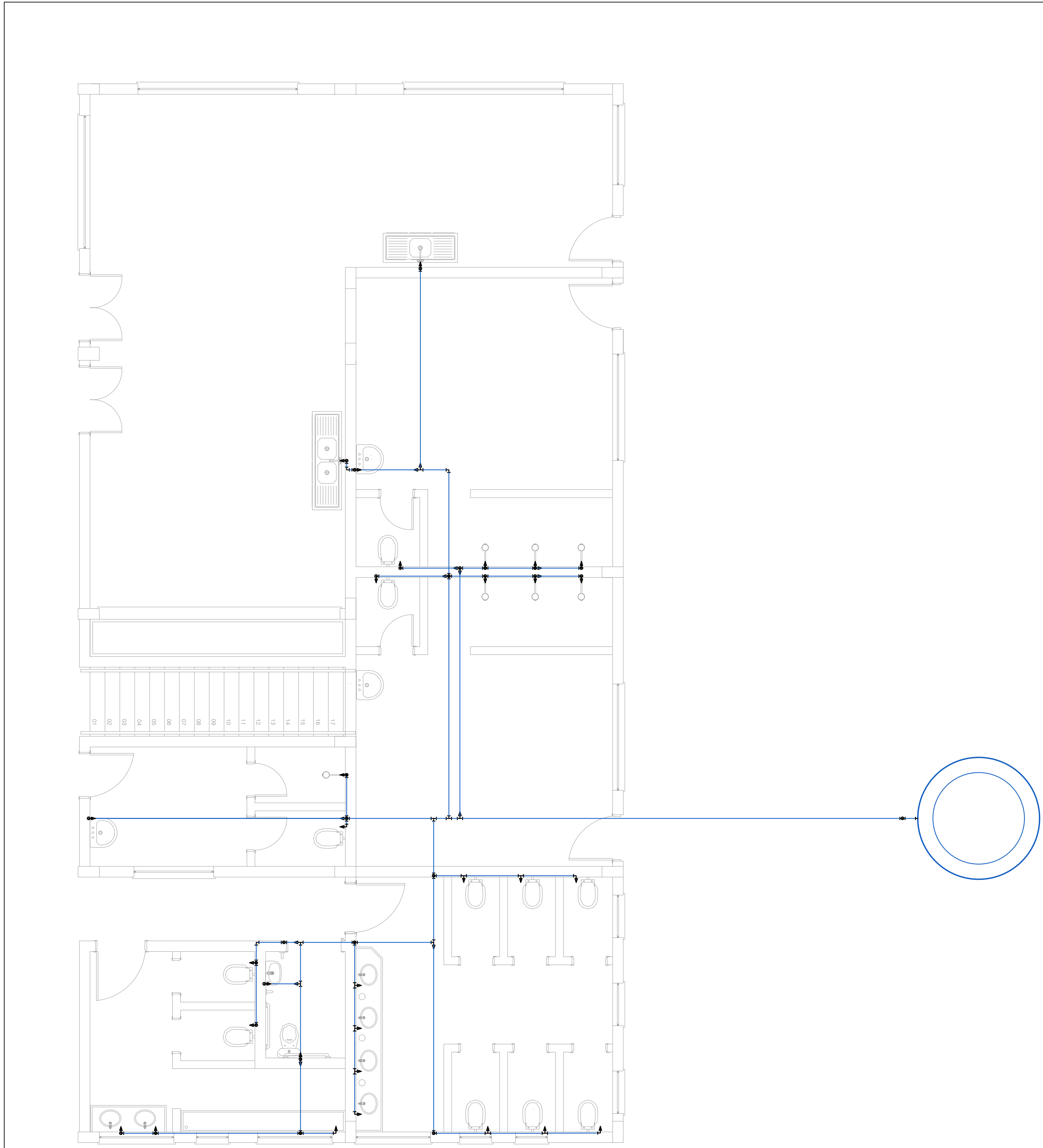
ABASTECIMENTO 17 escala: 1:50
