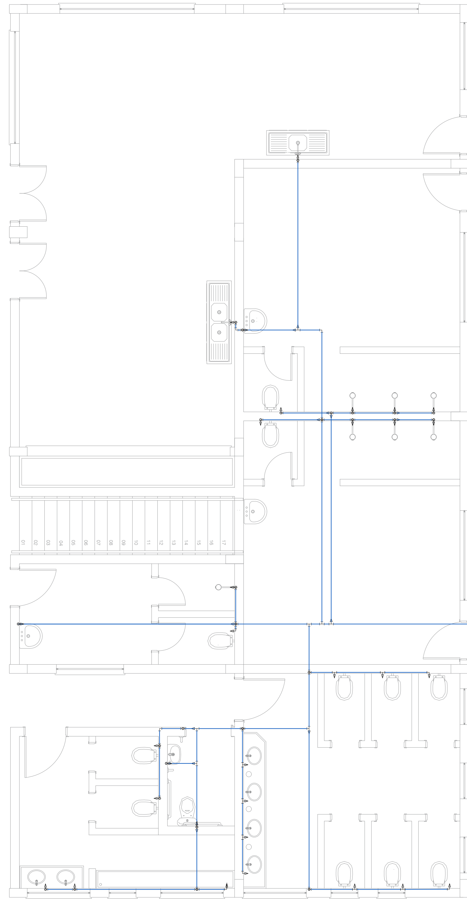
ABASTECIMENTO escala: 1:50
