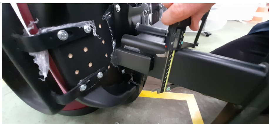
Fig. 14: Longarina 3 Lugares com Braços - L3 - Amostra fornecida
