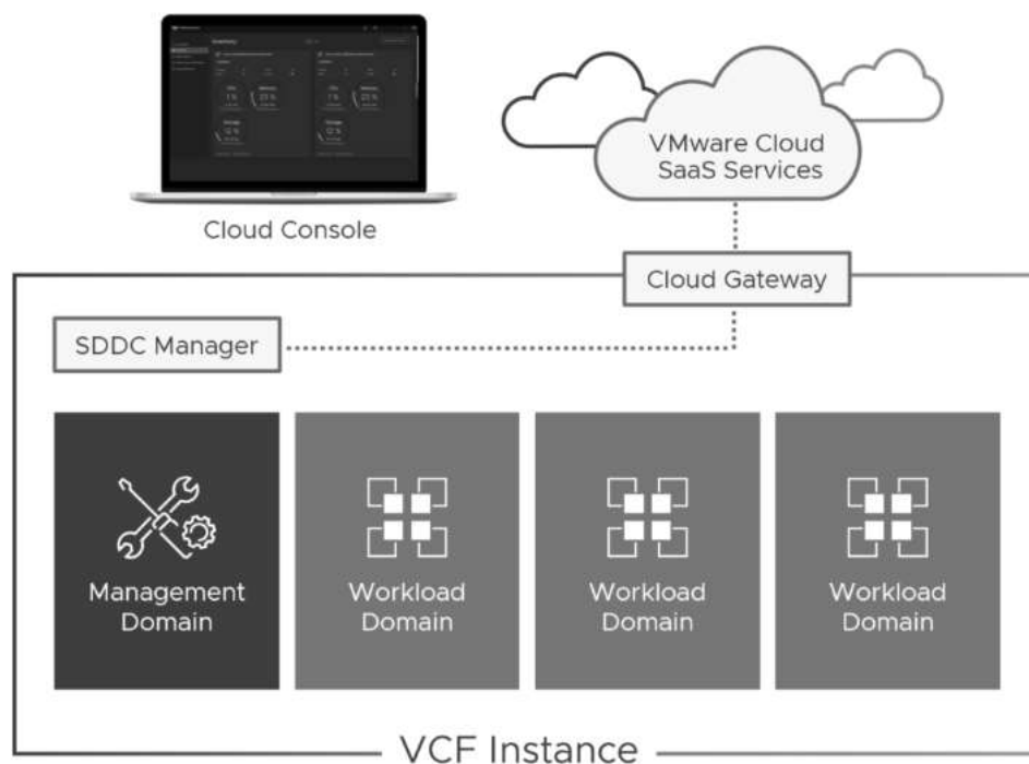
Figura 4 - Arquitetura do Produto VMware Cloud Foundation
