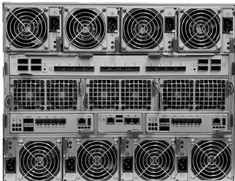
Figura 2 - Vista Traseira de Chassi Blade com 2 Módulos de Rede LAN, 1 Módulo Rede SAN, 8 Fontes de Alimentação e 6 Ventiladores
