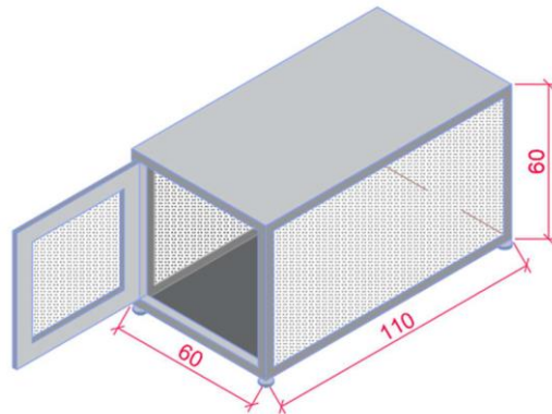
Figura 1- DIMENSÕES DO RACK QUE VAI FICAR SOBRE OS PALLETS
