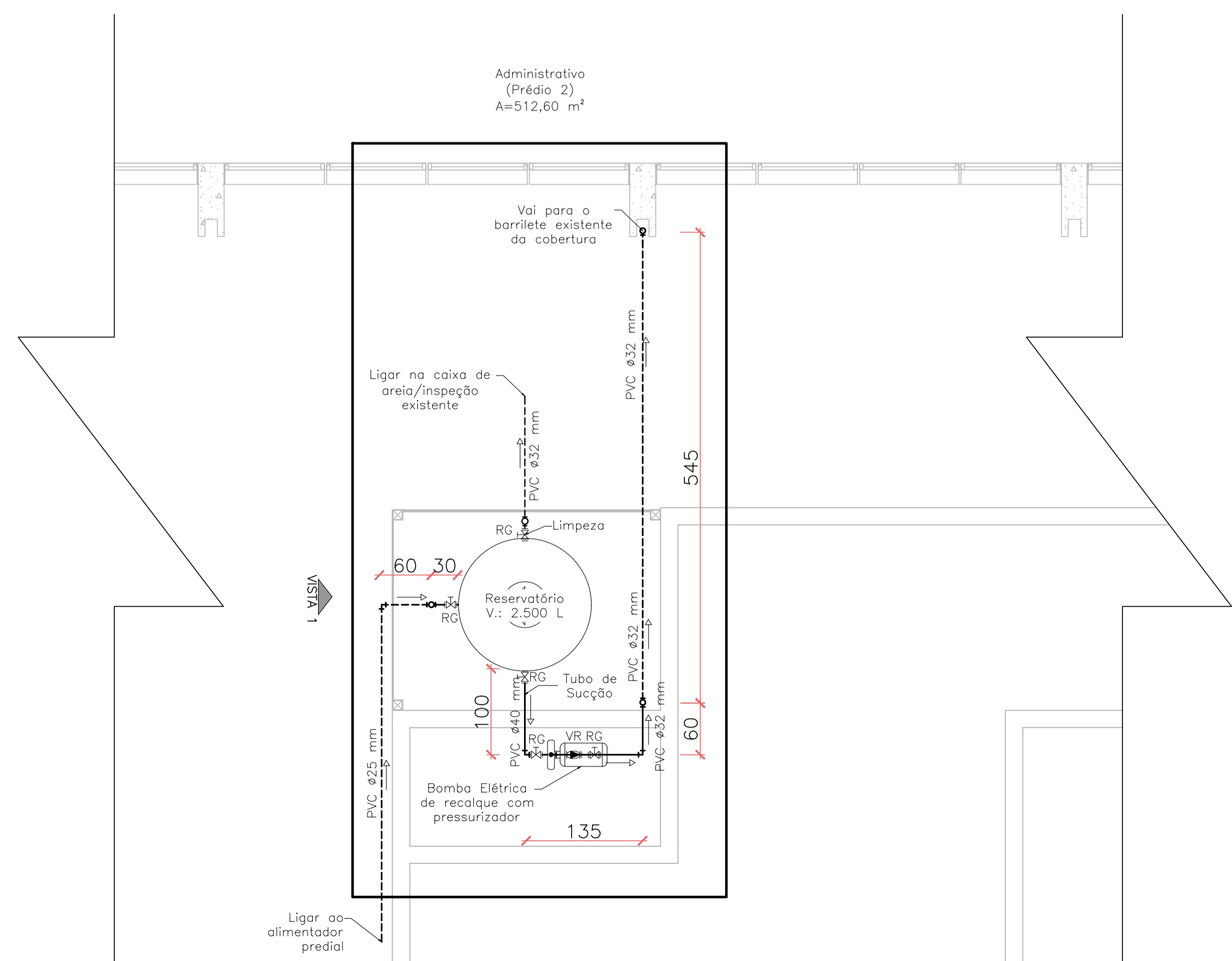
03 PLANTA BAIXA TÉRREO ESCALA: 1/50
