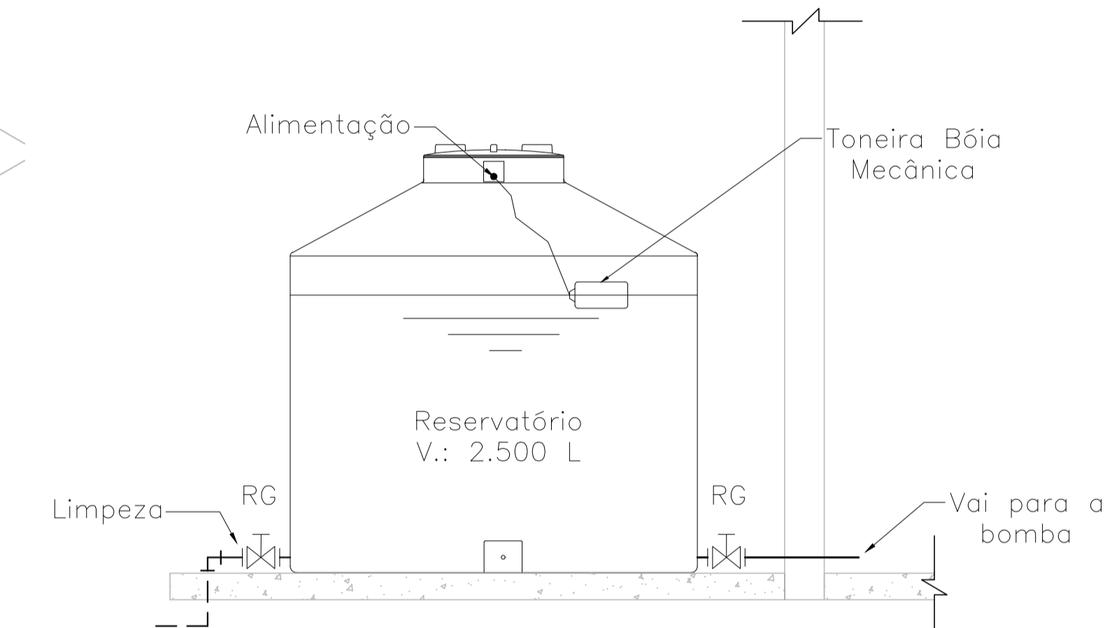
02 VISTA 01 ESCALA: 1/20
