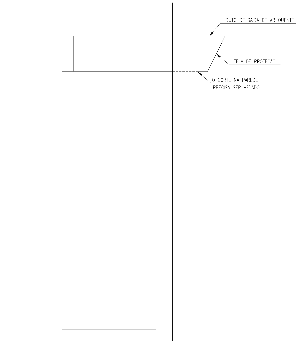
VISTA LATERAL
