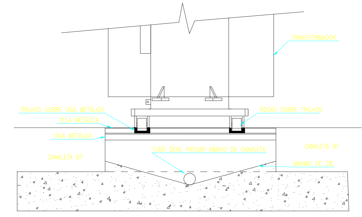
DETALHE 5 ESC. 1/20
