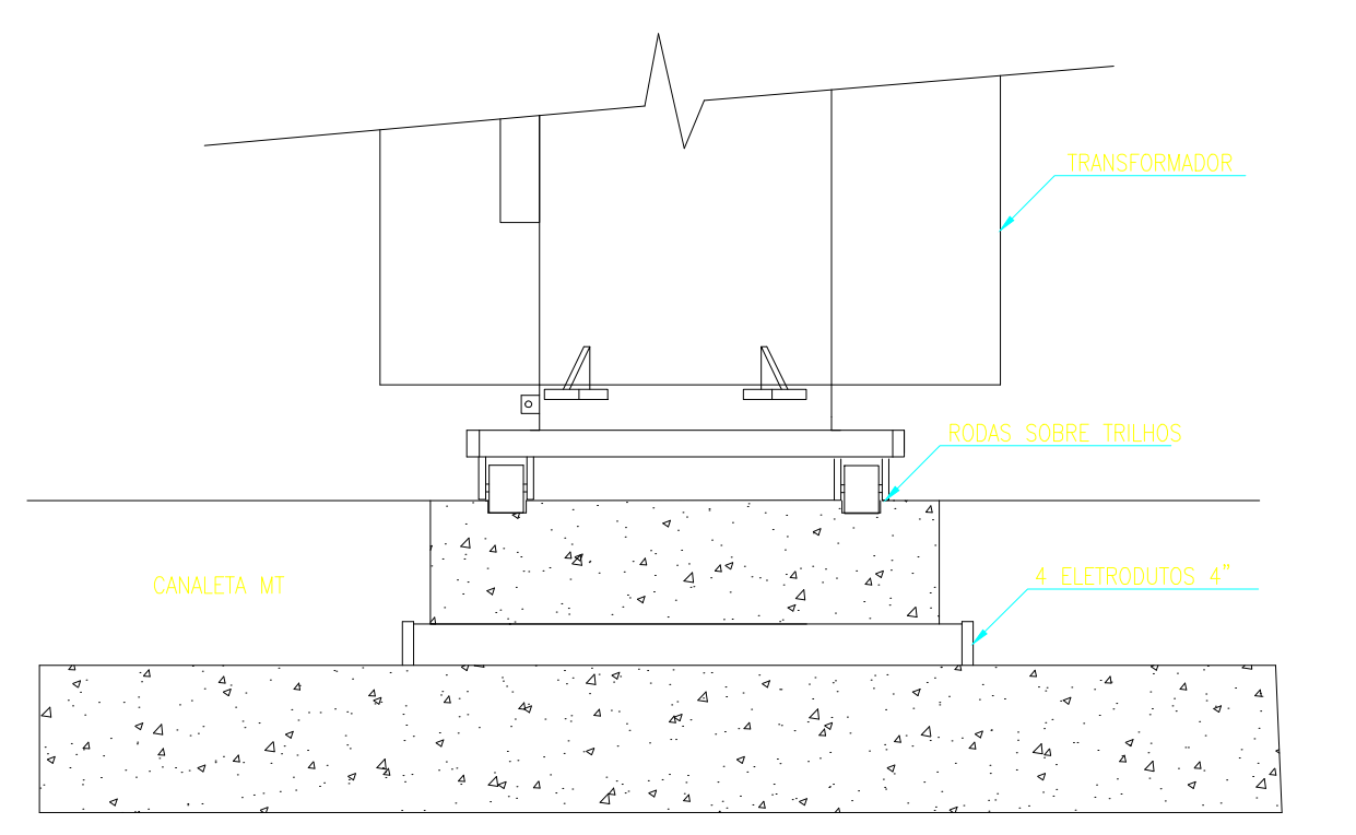
DETALHE 4 ESC. 1/20
