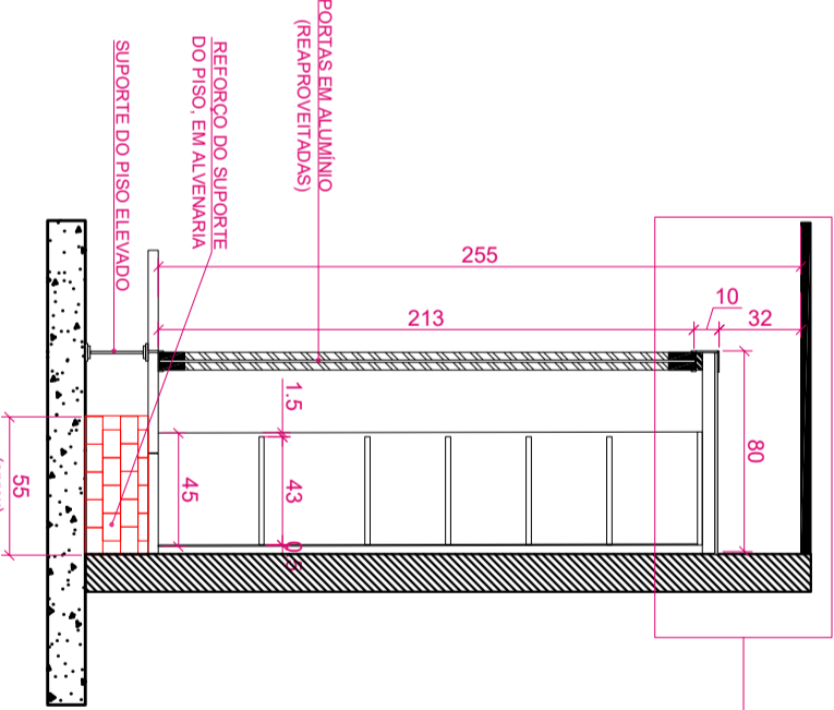
DETALHE ESTRUTURA PORTAS
