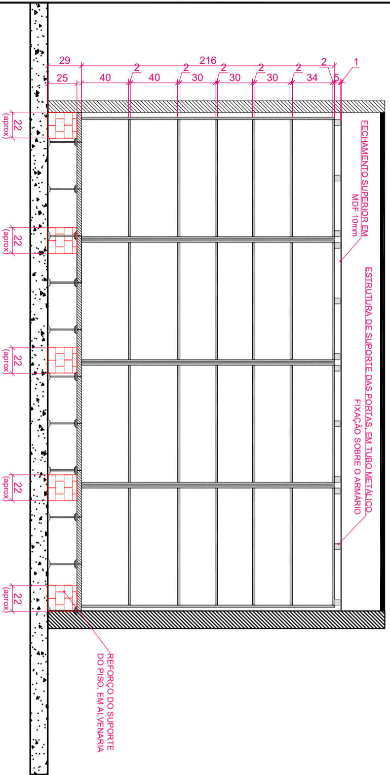
CORTE LONGITUDINAL
