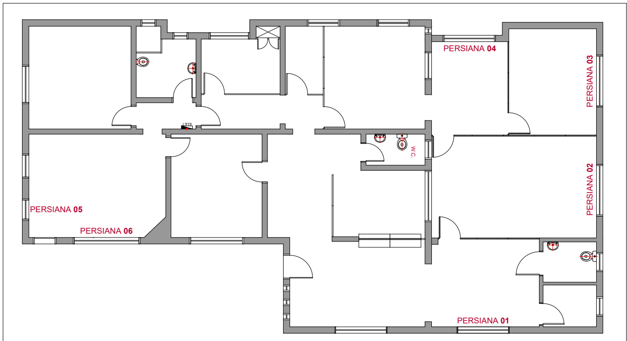
PLANTA BAIXA
