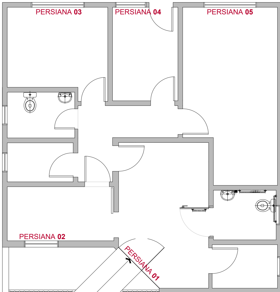
PLANTA BAIXA
