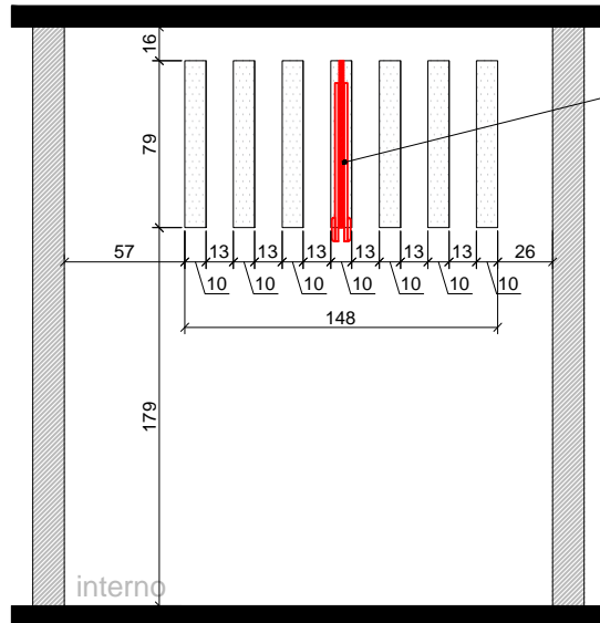
VISTA INTERNA
