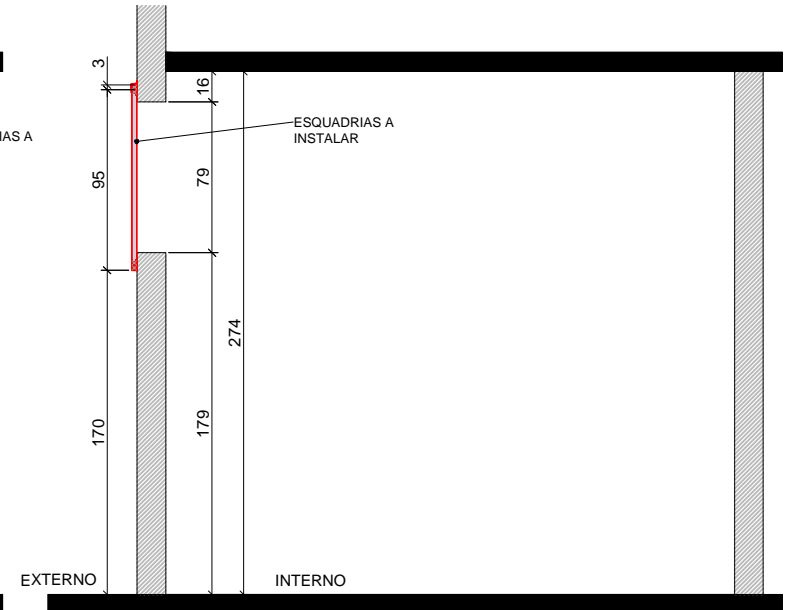
CORTE TRANSVERSAL
