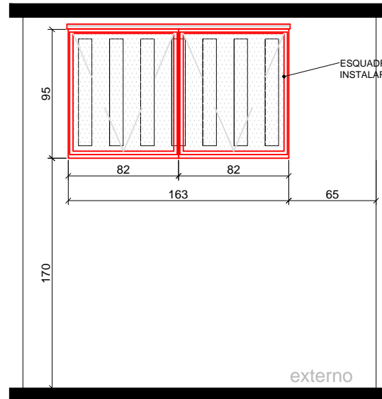
VISTA EXTERNA
